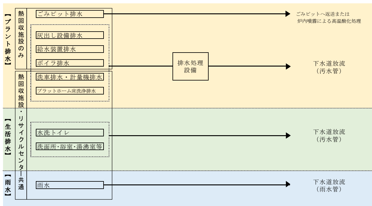
図 9-6 新施設で想定される排水処理フロー
