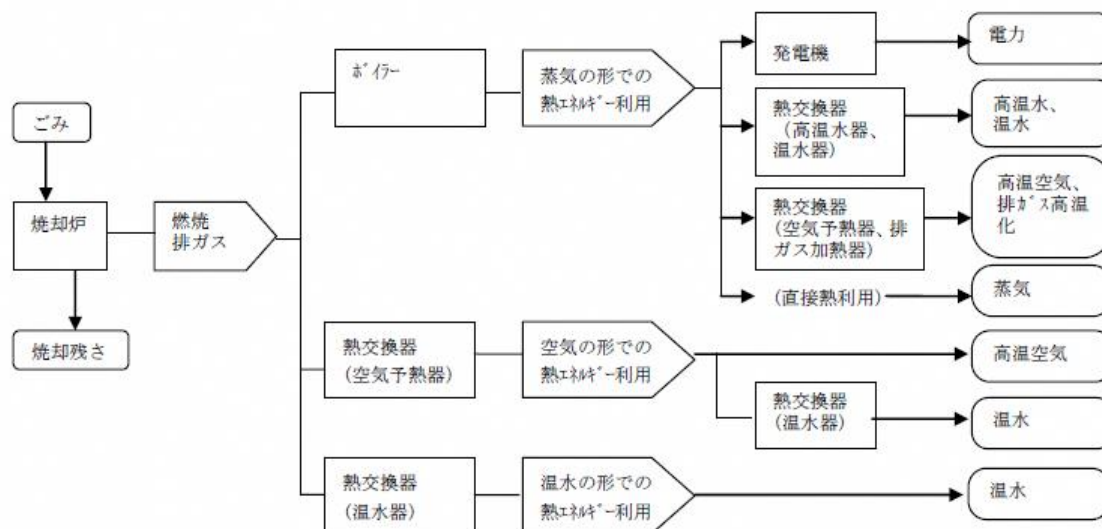
図 9-7 ごみ焼却排熱のエネルギー変換による熱利用形態
