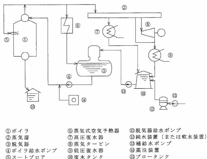
図 9-3 ボイラ設備フロー例
