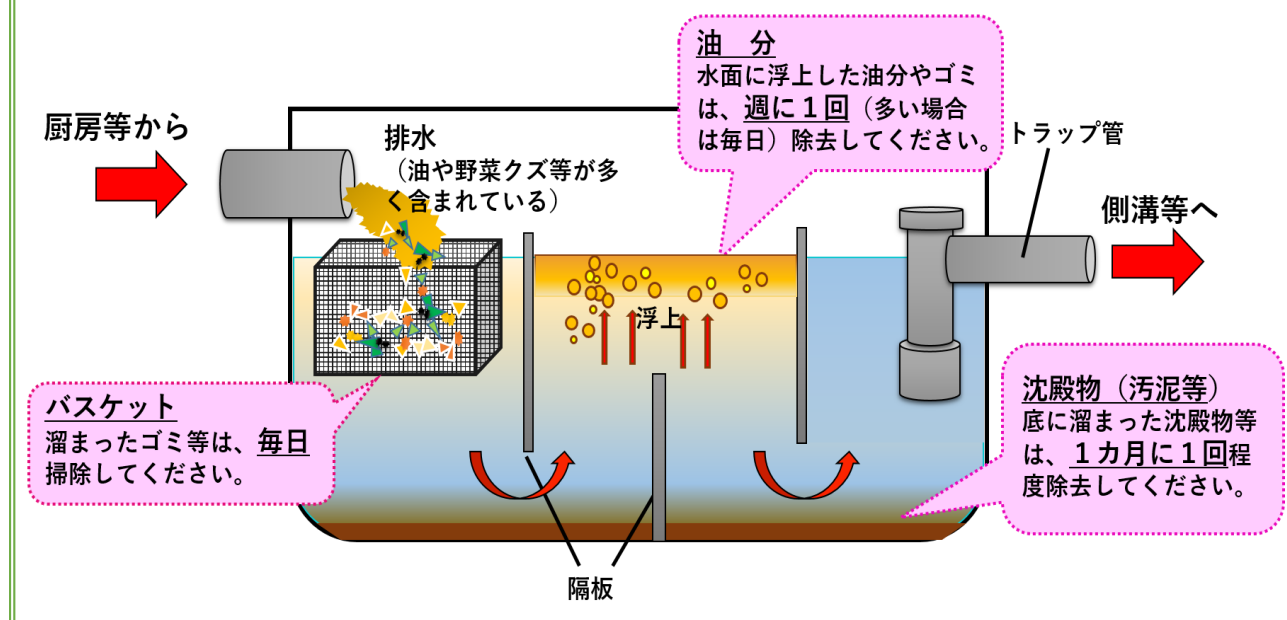
グリーストラップを横からみた図
