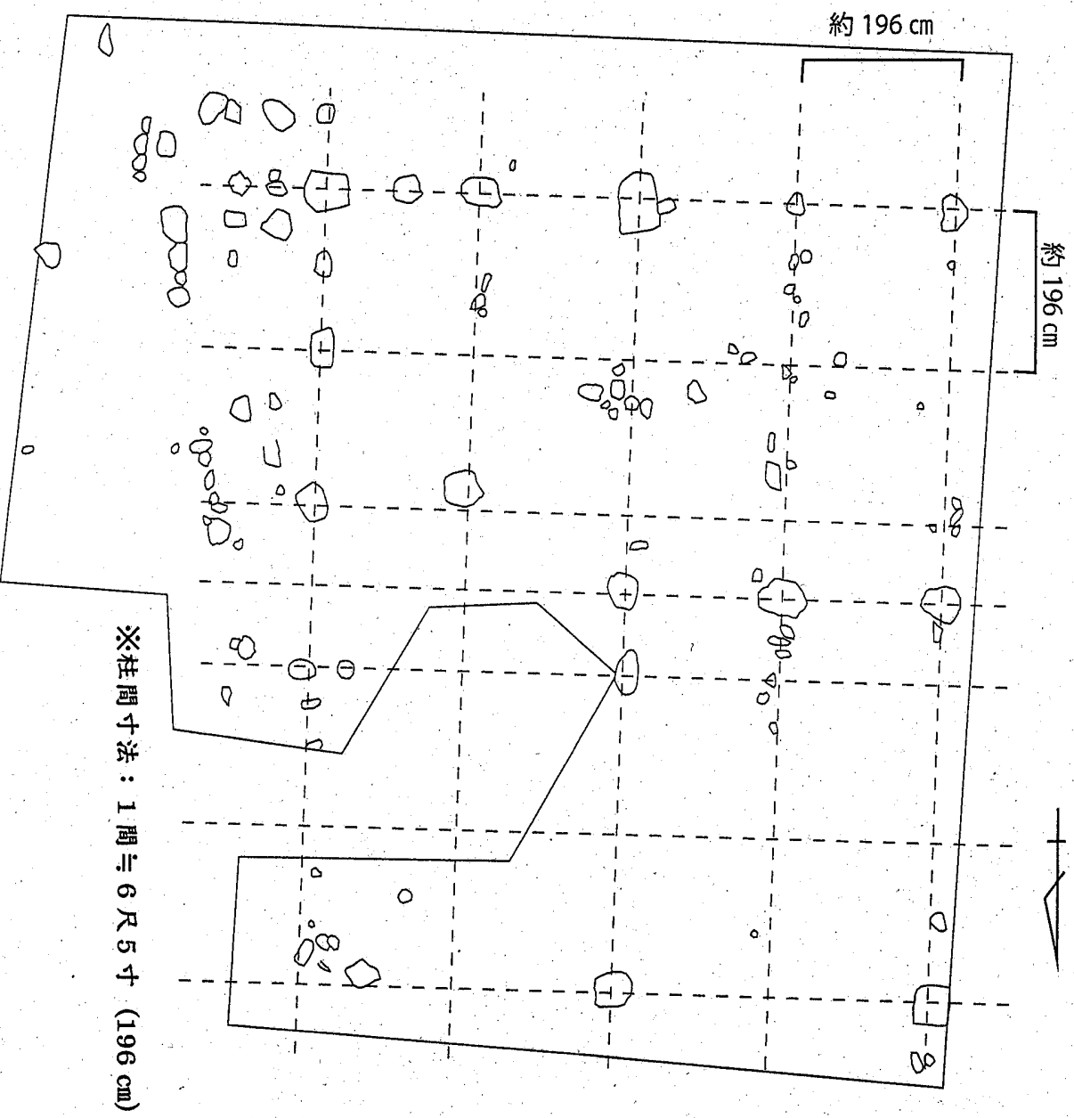
一宮城跡第2次発掘調査 (平成30年度) 平面概略図
