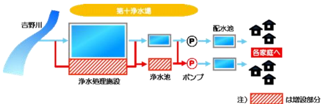
図3.12 第十浄水場基幹施設建設（イメージ）
