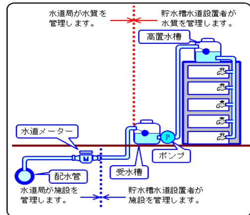
図 6.2 貯水槽水道の設備イメージと管理区分
